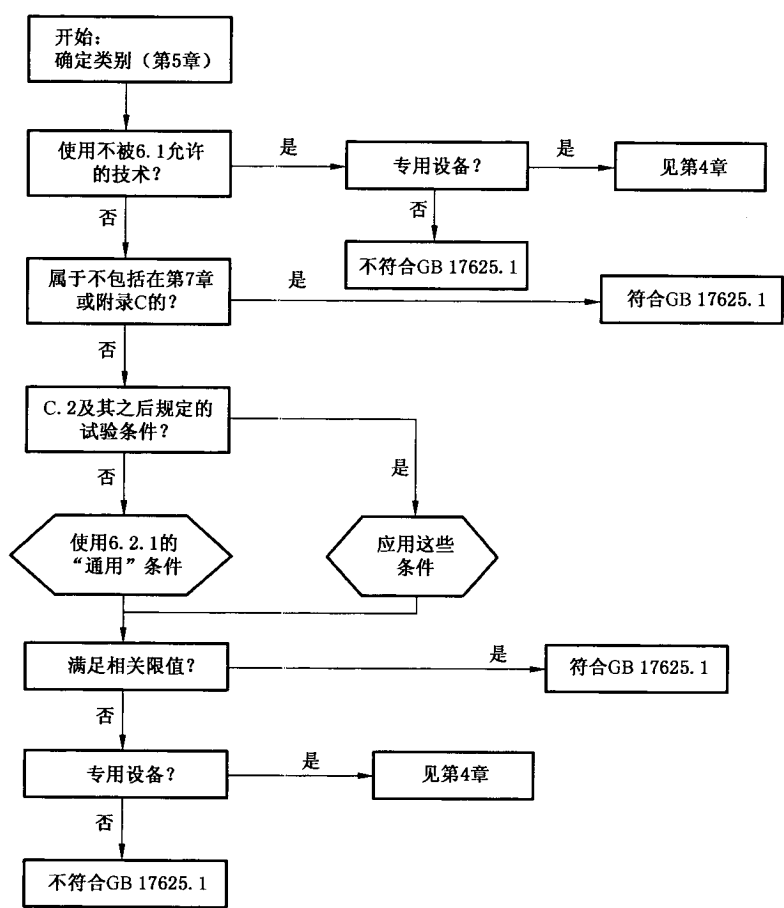
图 1 符合性确定流程图
